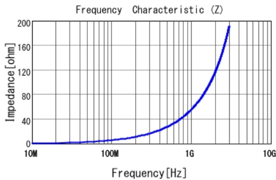
■ LQW15AN9N1G00 |Z|
