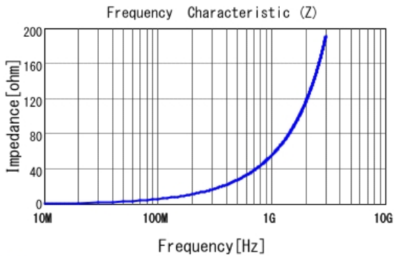
■ LQW15AN9N1H00 |Z|
