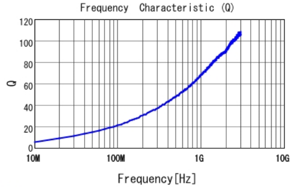
■ LQW15AN9N1H00 Q
