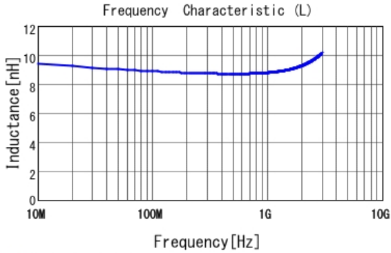
■ LQW15AN9N1H00 L
