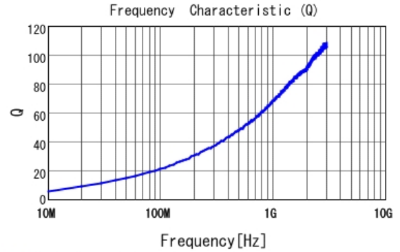
■ LQW15AN9N1J00 Q
