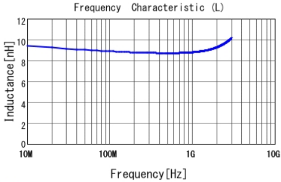
■ LQW15AN9N1J00 L
