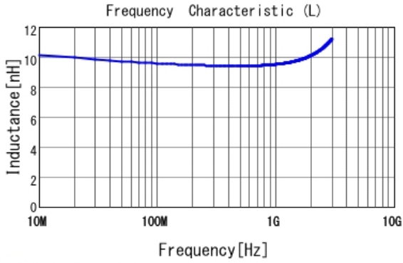
■ LQW15AN9N5G00 L
