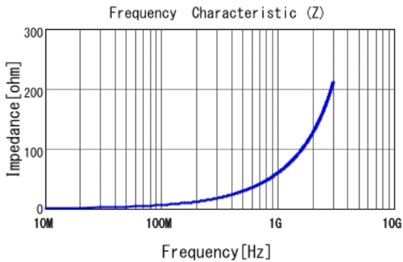
■ LQW15AN9N5G00 |Z|
