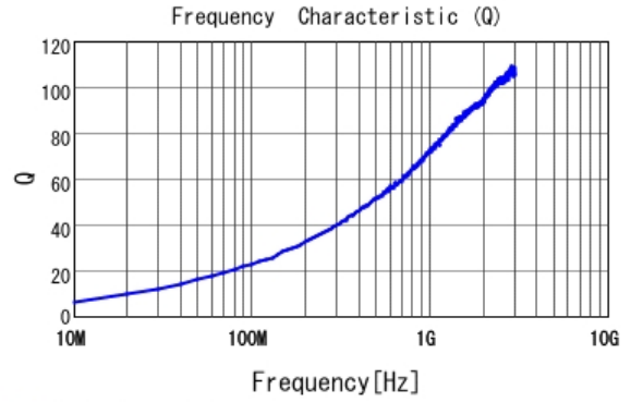
■ LQW15AN9N5G00 Q
