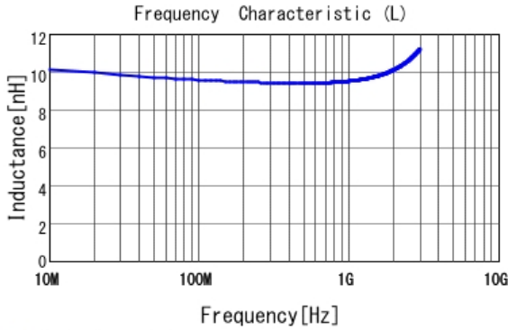
■ LQW15AN9N5H00 L
