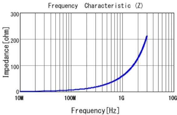
■ LQW15AN9N5H00 |Z|
