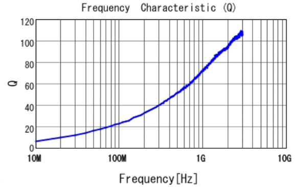
■ LQW15AN9N5H00 Q
