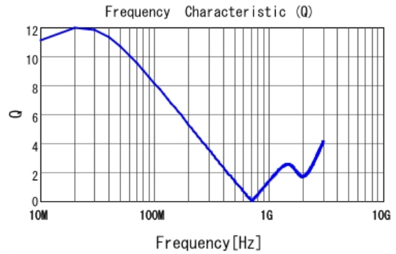
■ LQW15CA1R0K00 Q
