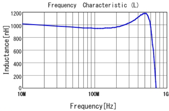
■ LQW15CA1R0K00 L
