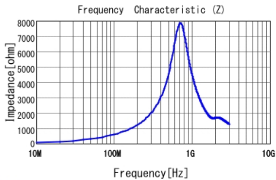
■ LQW15CA1R0K00 |Z|
