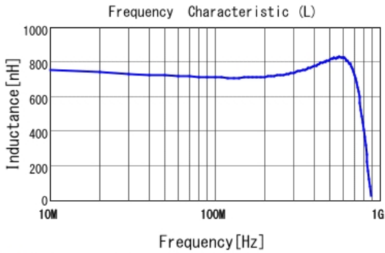
■ LQW15CAR73J00 L
