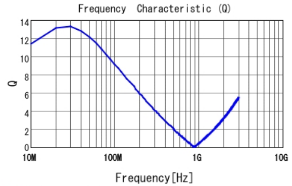
■ LQW15CAR73J00 Q
