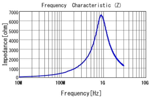
■ LQW15CAR73J00 |Z|
