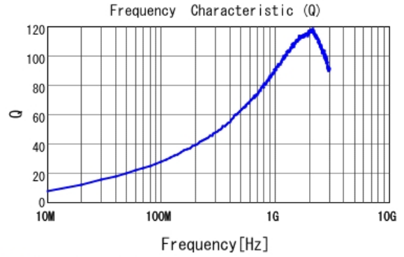
■ LQW18AN12NG00 Q
