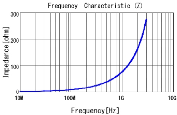
■ LQW18AN12NG00 |Z|
