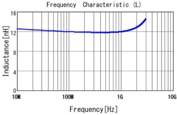
■ LQW18AN12NG00 L
