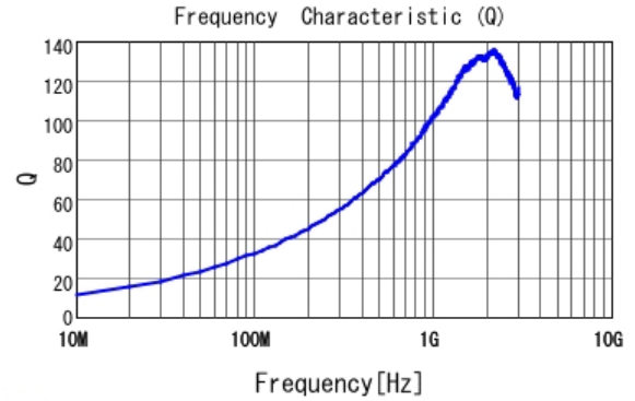
■ LQW18AN12NJ10 Q
