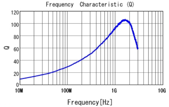
■ LQW18AN15NJ00 Q
