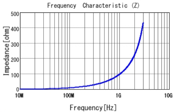
■ LQW18AN15NJ00 |Z|
