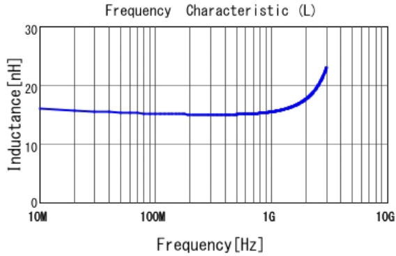
■ LQW18AN15NJ00 L
