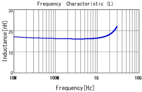
■ LQW18AN16NG00 L
