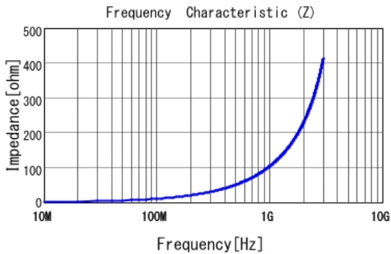
■ LQW18AN16NG00 |Z|
