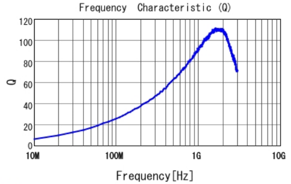
■ LQW18AN16NG00 Q
