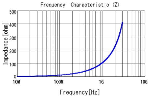
■ LQW18AN16NJ00 |Z|
