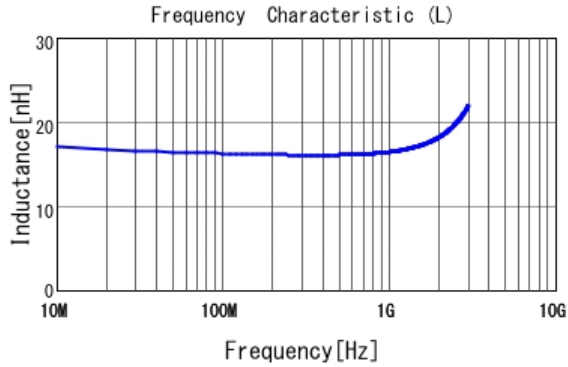
■ LQW18AN16NJ00 L
