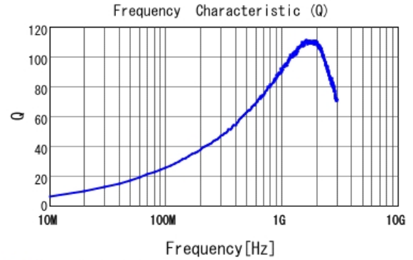
■ LQW18AN16NJ00 Q
