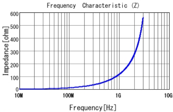
■ LQW18AN18NG00 |Z|
