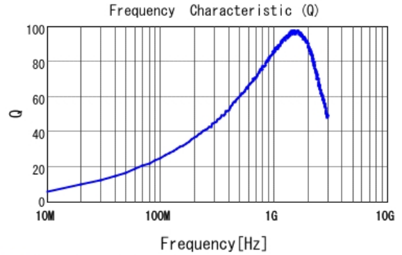
■ LQW18AN18NG00 Q
