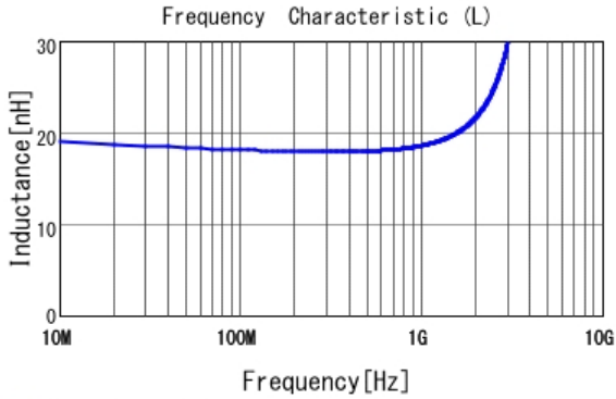
■ LQW18AN18NG00 L
