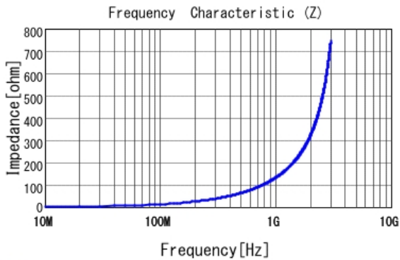
■ LQW18AN20NG00 |Z|
