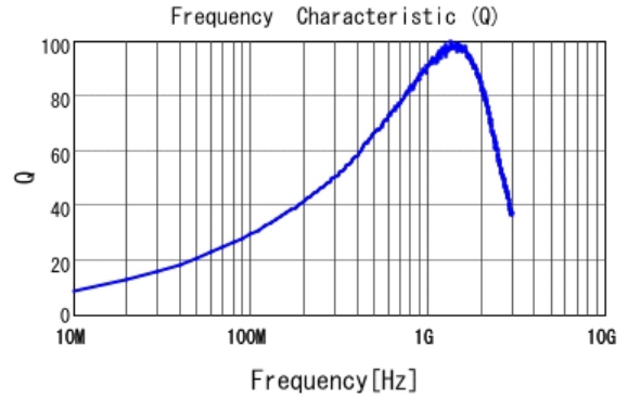
■ LQW18AN20NG00 Q
