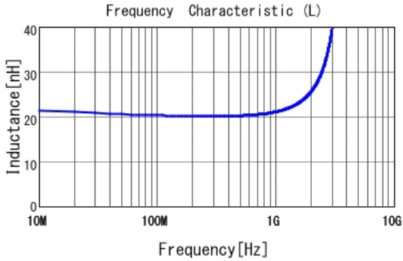
■ LQW18AN20NG00 L
