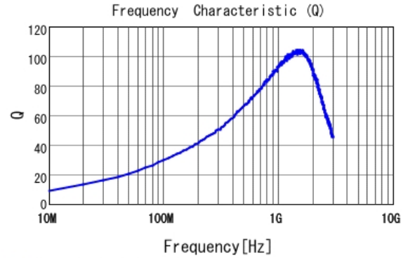
■ LQW18AN22NJ00 Q
