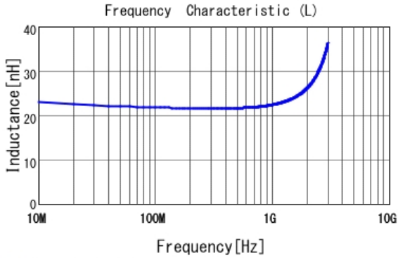
■ LQW18AN22NJ00 L
