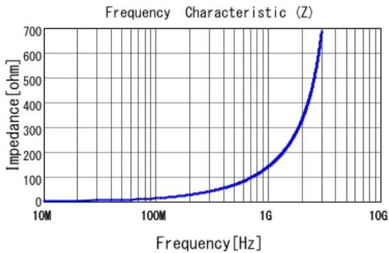
■ LQW18AN22NJ00 |Z|
