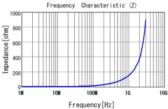
■ LQW18AN23NG80 |Z|
