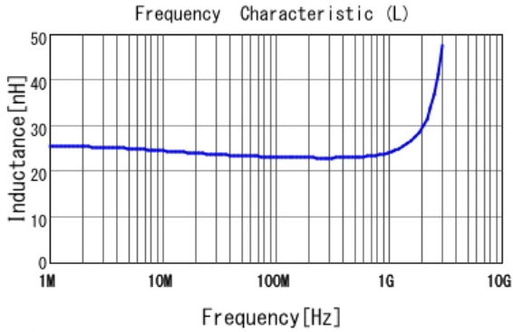
■ LQW18AN23NG80 L
