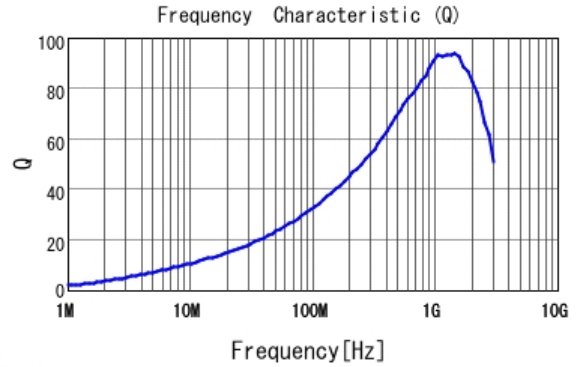
■ LQW18AN23NG80 Q
