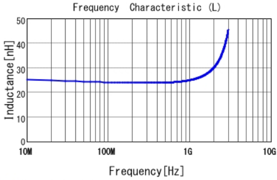
■ LQW18AN24NG00 L
