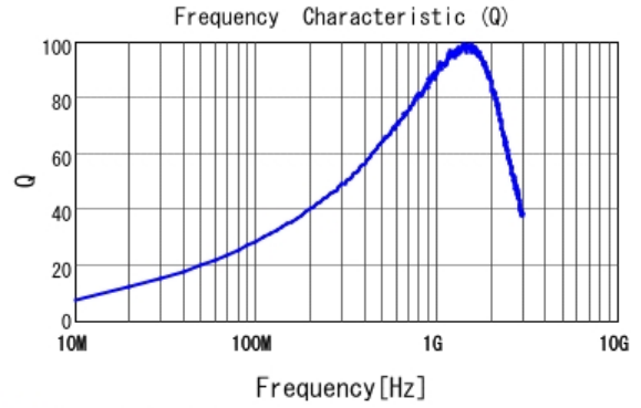
■ LQW18AN24NG00 Q
