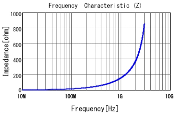
■ LQW18AN24NG00 |Z|
