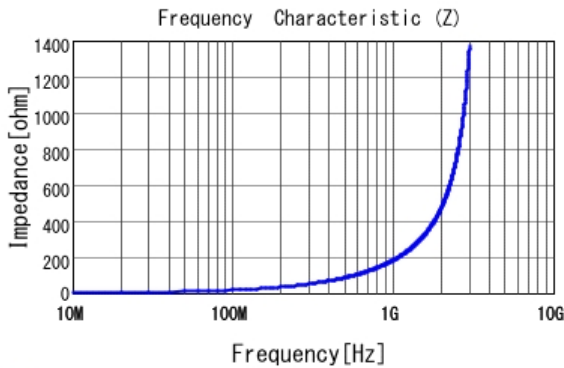
■ LQW18AN27NG00 |Z|
