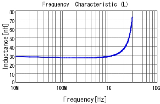
■ LQW18AN27NG00 L
