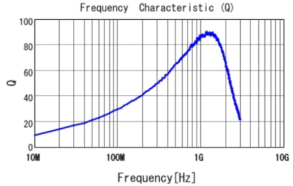
■ LQW18AN27NG00 Q
