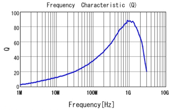
■ LQW18AN28NJ8Z Q
