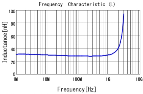
■ LQW18AN28NJ8Z L
