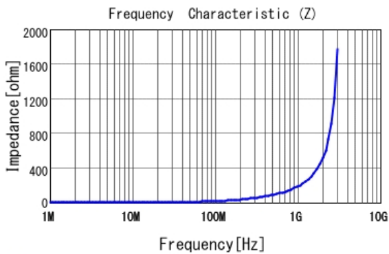
■ LQW18AN28NJ8Z |Z|
