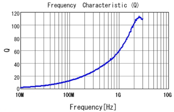
■ LQW18AN2N2C80 Q
