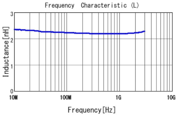
■ LQW18AN2N2C80 L
