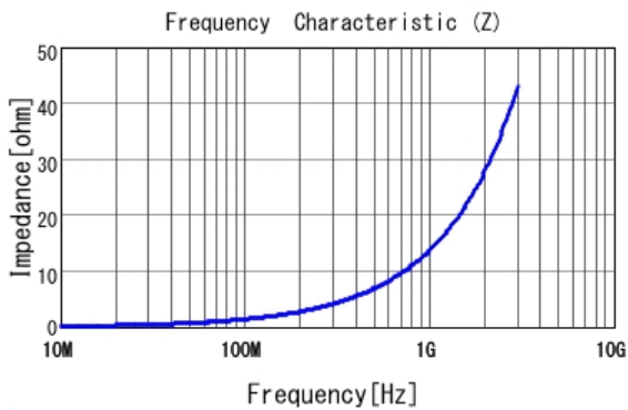
■ LQW18AN2N2C80 |Z|
