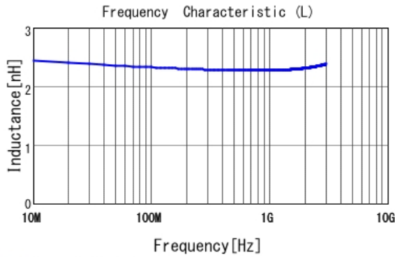
■ LQW18AN2N2D0Z L
