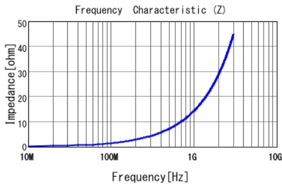
■ LQW18AN2N2D0Z |Z|
