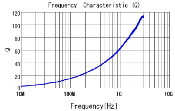
■ LQW18AN2N2D0Z Q
