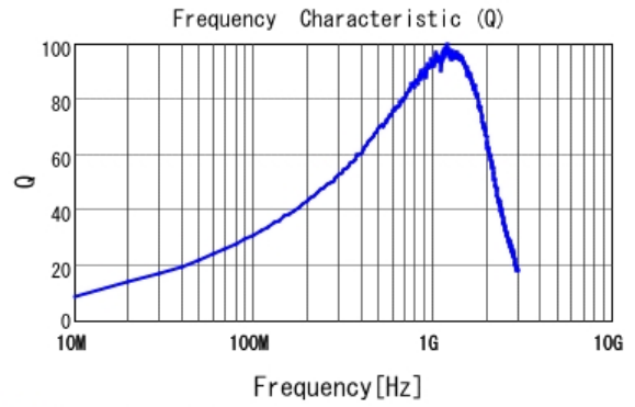
■ LQW18AN36NG00 Q
