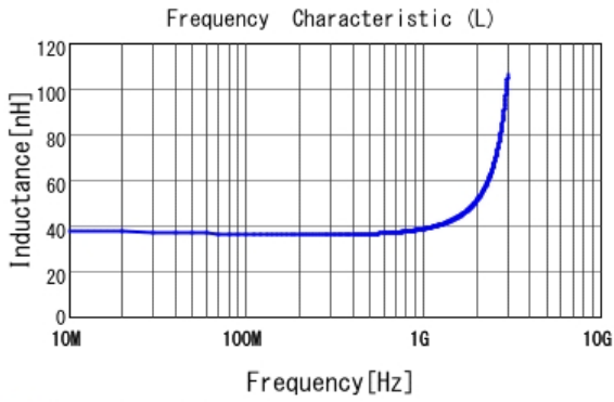
■ LQW18AN36NG00 L
