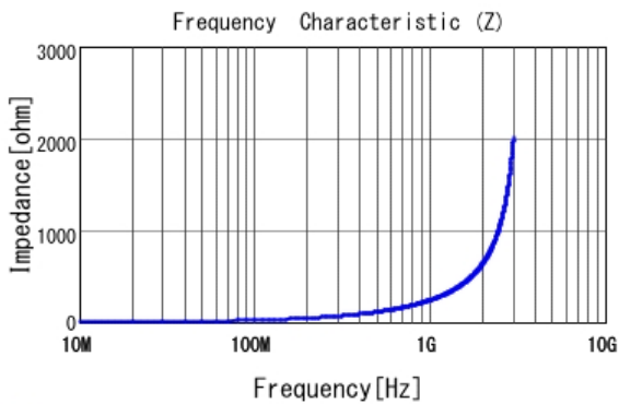
■ LQW18AN36NG00 |Z|
