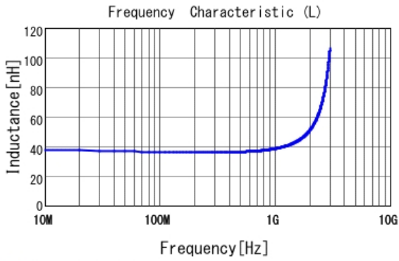
■ LQW18AN36NJ00 L
