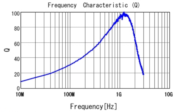
■ LQW18AN36NJ00 Q
