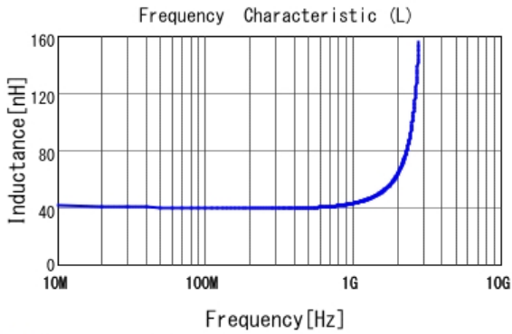
■ LQW18AN39NG00 L
