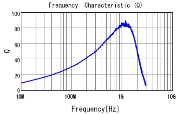
■ LQW18AN39NG00 Q
