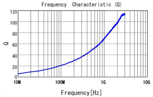
■ LQW18AN3N6C00 Q
