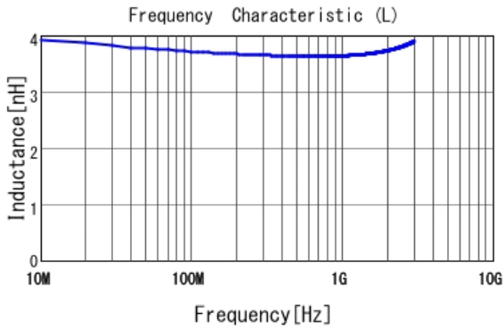
■ LQW18AN3N6C00 L
