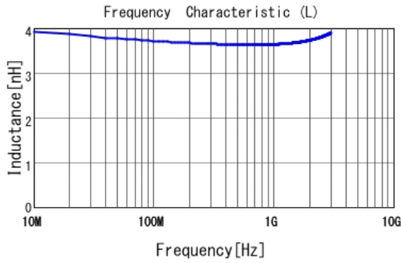
■ LQW18AN3N6C0Z L
