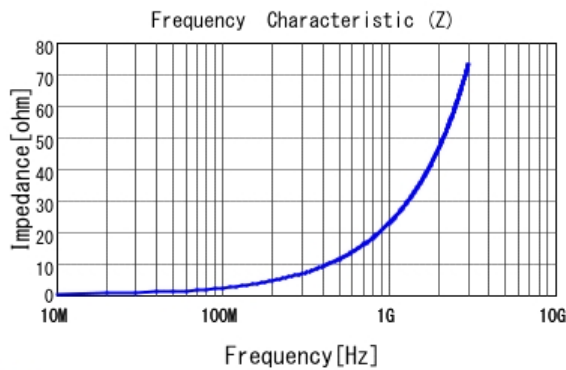
■ LQW18AN3N6C0Z |Z|
