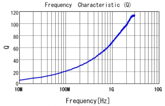
■ LQW18AN3N6C0Z Q
