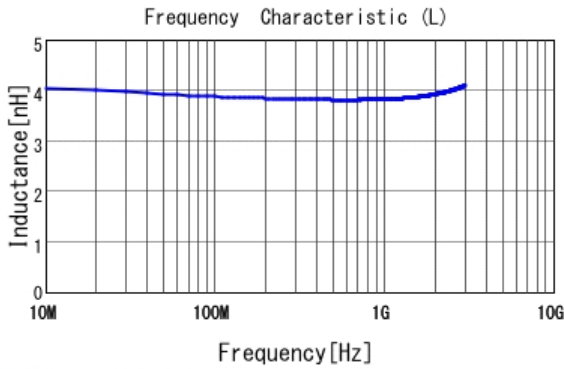
■ LQW18AN3N9C00 L
