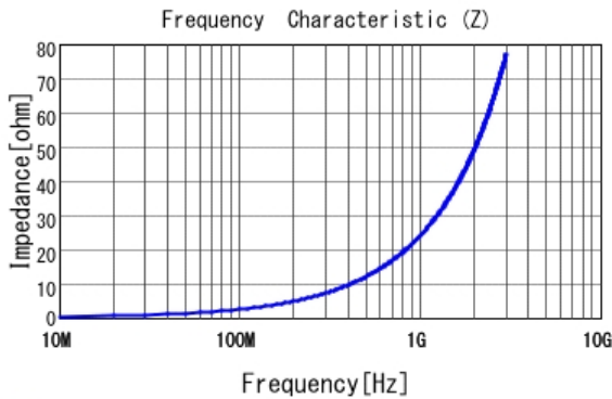
■ LQW18AN3N9C00 |Z|
