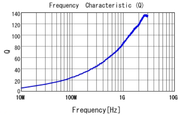
■ LQW18AN3N9C00 Q
