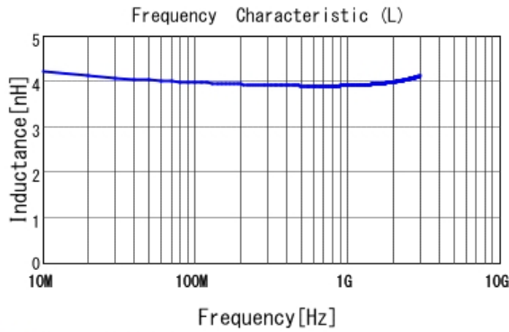
■ LQW18AN3N9C10 L
