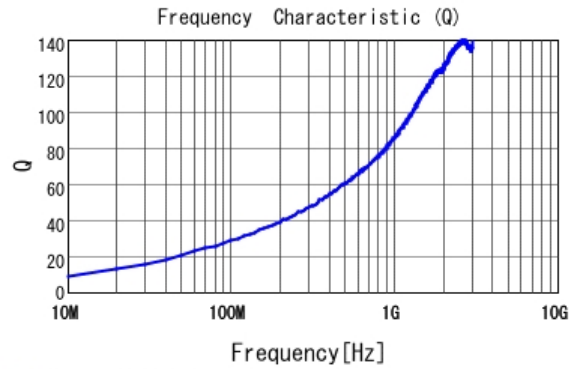
■ LQW18AN3N9C10 Q
