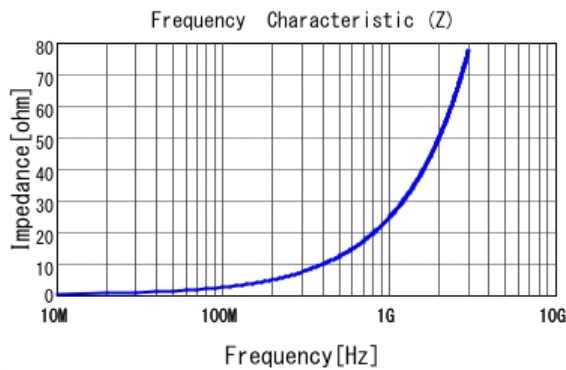
■ LQW18AN3N9C10 |Z|
