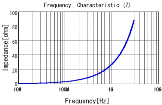
■ LQW18AN4N3C00 |Z|
