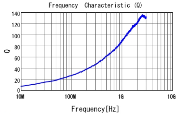
■ LQW18AN4N3C00 Q
