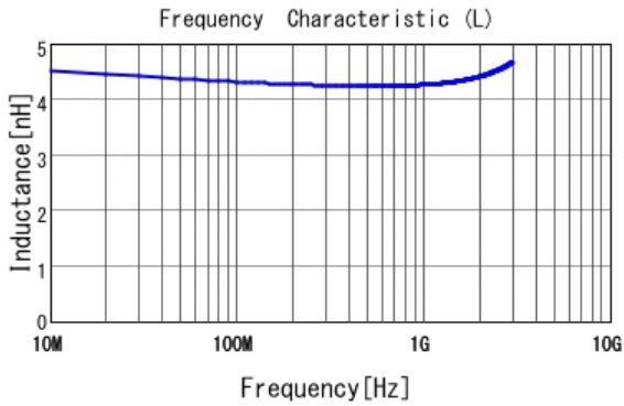
■ LQW18AN4N3C00 L
