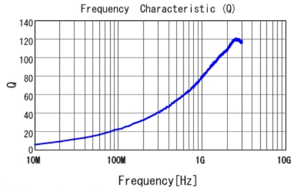
■ LQW18AN4N7D00 Q
