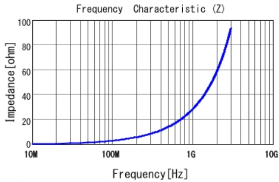
■ LQW18AN4N7D00 |Z|
