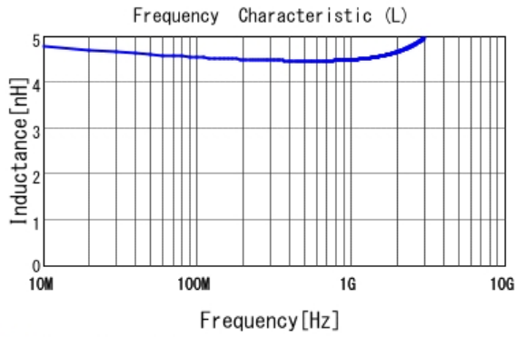
■ LQW18AN4N7D00 L
