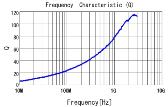
■ LQW18AN4N7G80 Q
