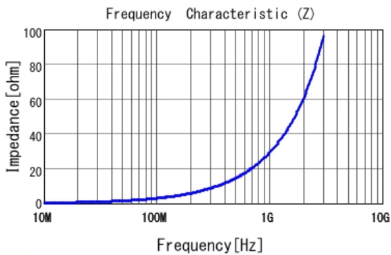
■ LQW18AN4N7G80 |Z|
