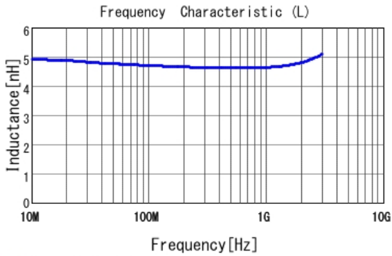
■ LQW18AN4N7G80 L
