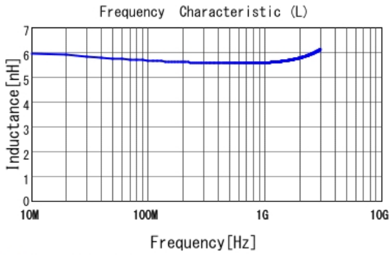
■ LQW18AN5N6C00 L
