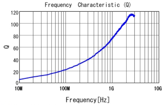
■ LQW18AN5N6C00 Q
