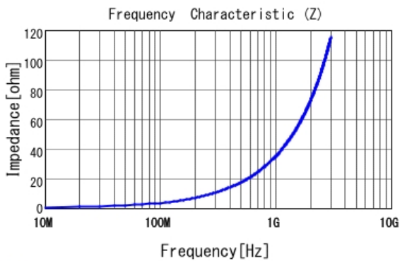
■ LQW18AN5N6C00 |Z|
