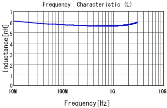
■ LQW18AN5N6D10 L
