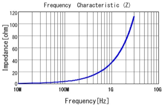
■ LQW18AN5N6D10 |Z|
