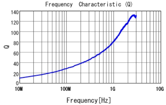
■ LQW18AN5N6D10 Q
