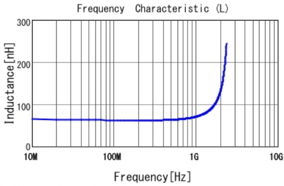
■ LQW18AN62NJ00 L
