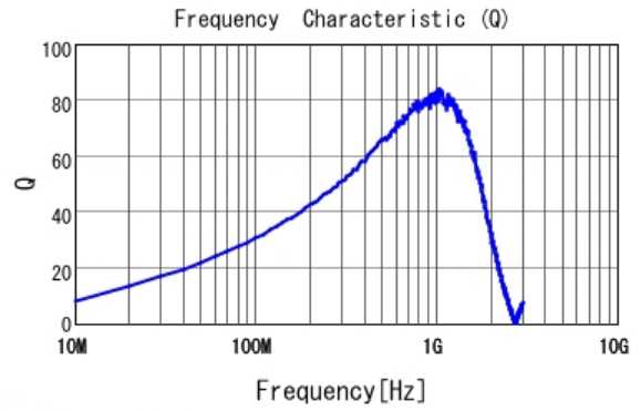
■ LQW18AN62NJ00 Q
