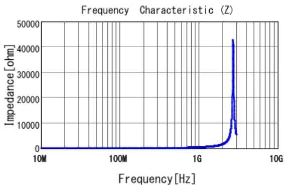
■ LQW18AN62NJ00 |Z|
