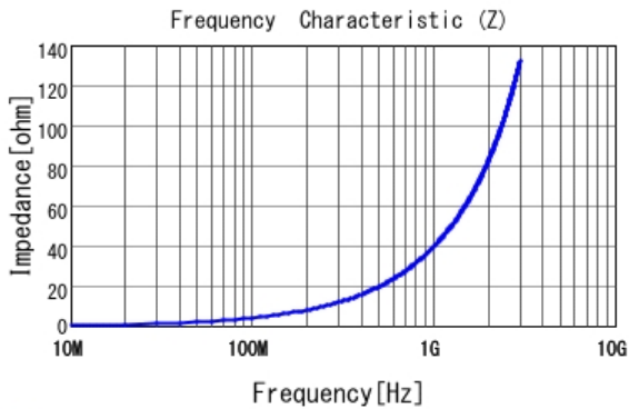
■ LQW18AN6N2C00 |Z|
