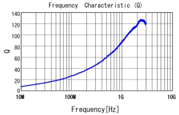
■ LQW18AN6N2C00 Q
