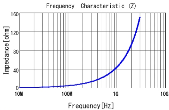
■ LQW18AN6N8C00 |Z|
