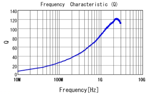
■ LQW18AN6N8C00 Q
