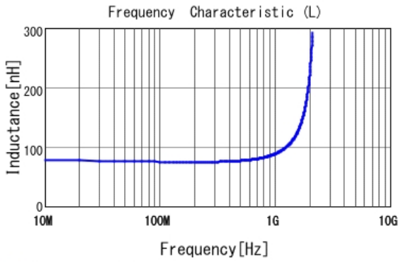
■ LQW18AN75NG00 L
