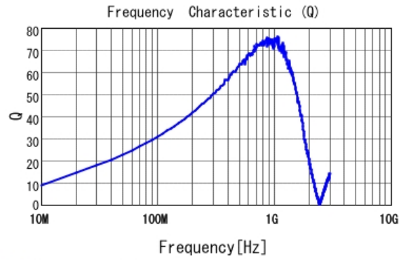
■ LQW18AN75NG00 Q
