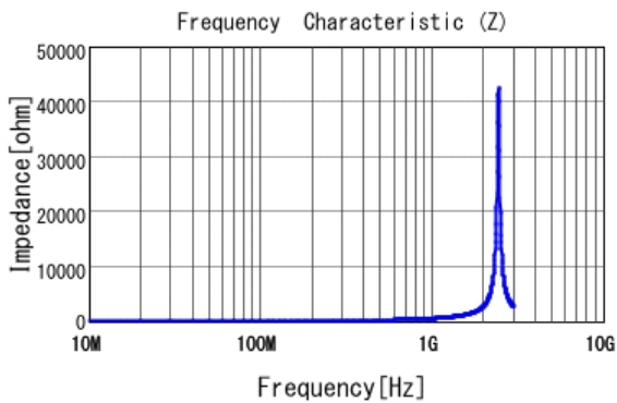
■ LQW18AN75NG00 |Z|
