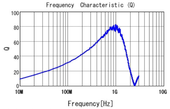
■ LQW18AN82NG00 Q
