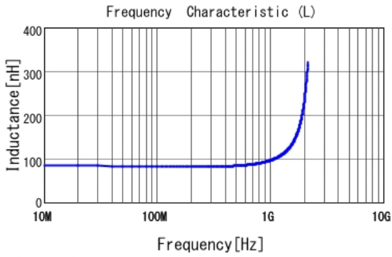
■ LQW18AN82NG00 L
