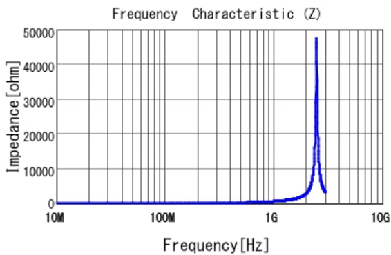
■ LQW18AN82NG00 |Z|
