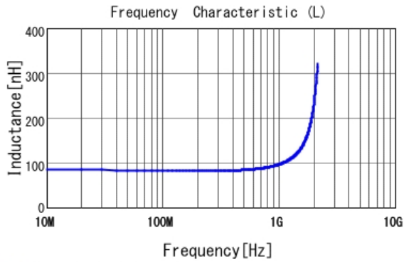
■ LQW18AN82NJ00 L
