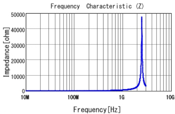
■ LQW18AN82NJ00 |Z|
