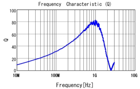
■ LQW18AN82NJ00 Q
