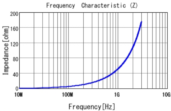
■ LQW18AN8N2D00 |Z|
