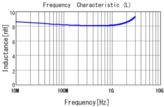
■ LQW18AN8N2D00 L
