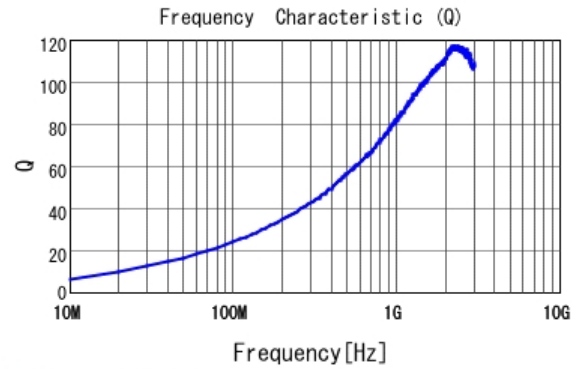
■ LQW18AN8N2D00 Q
