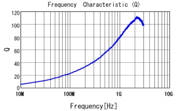
■ LQW18AN8N7C00 Q
