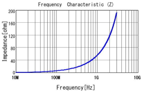
■ LQW18AN8N7C00 |Z|
