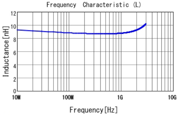
■ LQW18AN8N7C00 L
