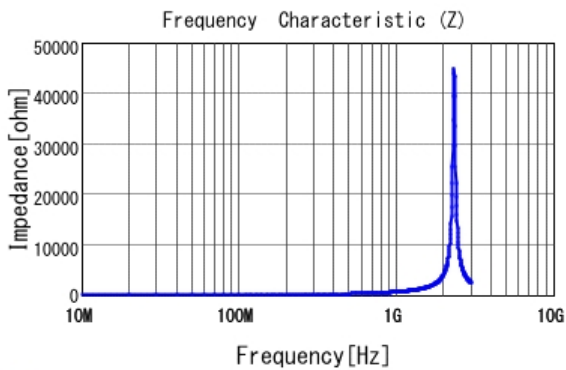
■ LQW18AN91NG0Z |Z|
