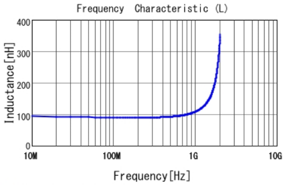
■ LQW18AN91NG0Z L
