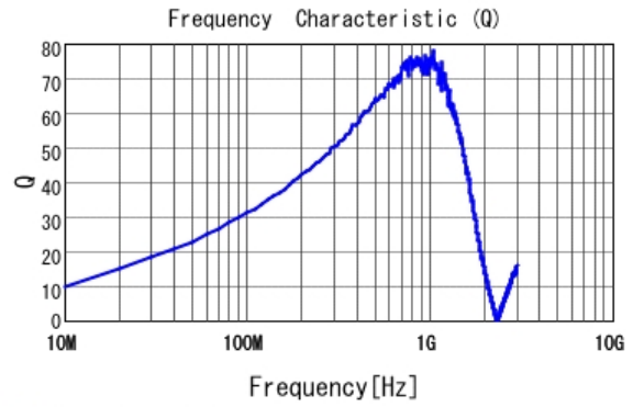
■ LQW18AN91NG0Z Q
