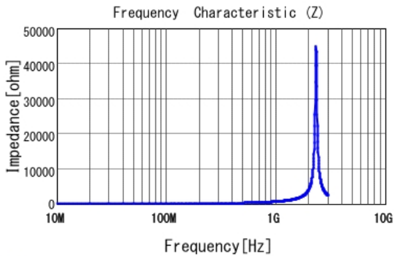
■ LQW18AN91NJ00 |Z|
