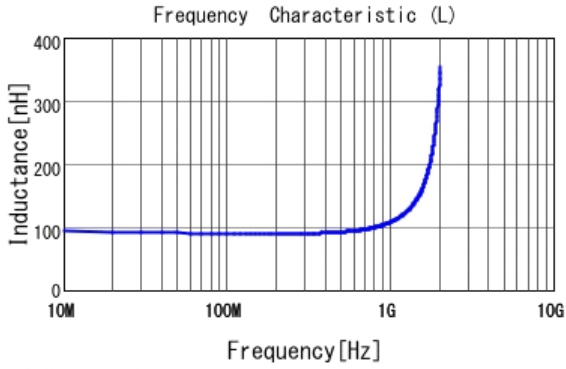
■ LQW18AN91NJ00 L
