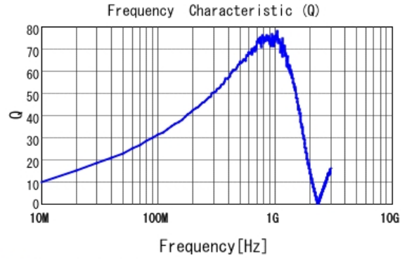
■ LQW18AN91NJ00 Q
