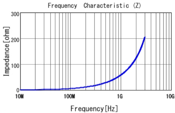
■ LQW18AN9N1C00 |Z|
