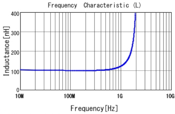
■ LQW18ANR10J00 L
