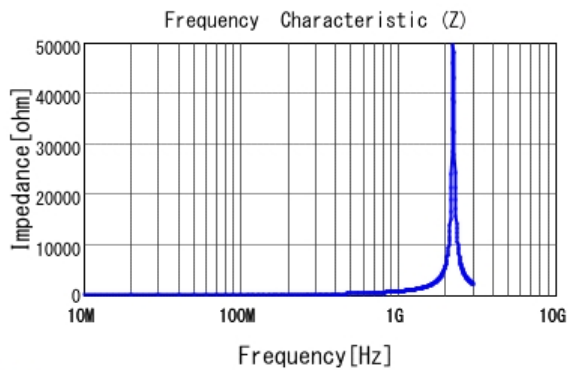
■ LQW18ANR10J00 |Z|
