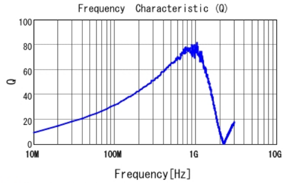
■ LQW18ANR10J00 Q
