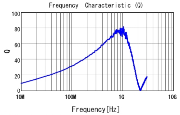
■ LQW18ANR10J0Z Q
