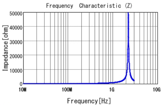
■ LQW18ANR10J0Z |Z|
