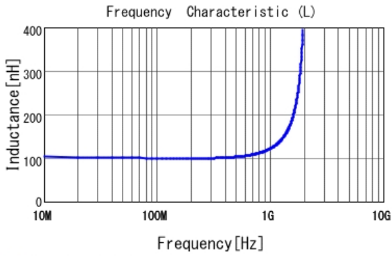
■ LQW18ANR10J0Z L
