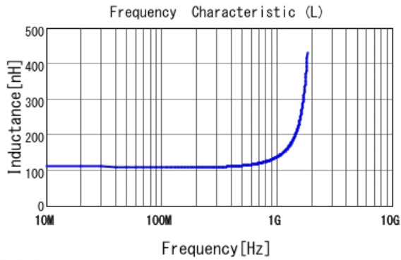
■ LQW18ANR11G00 L
