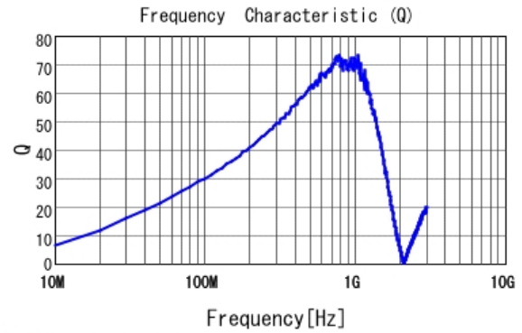
■ LQW18ANR11G00 Q
