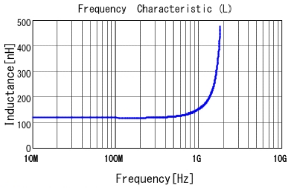
■ LQW18ANR12G00 L
