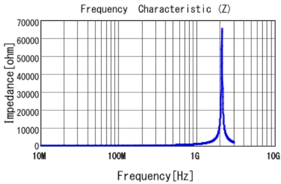
■ LQW18ANR12G00 |Z|
