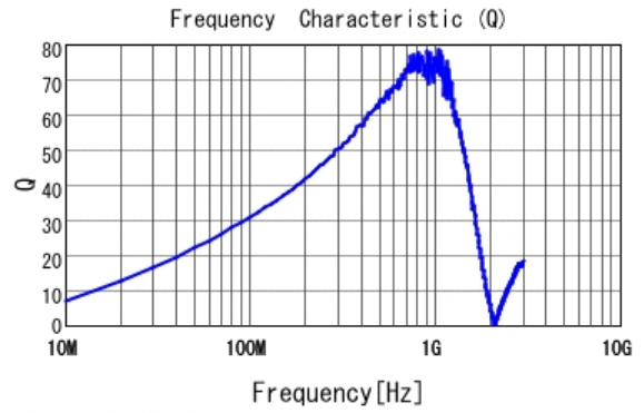
■ LQW18ANR12G00 Q
