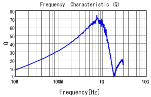
■ LQW18ANR15G00 Q
