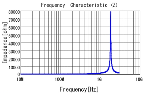
■ LQW18ANR15G00 |Z|
