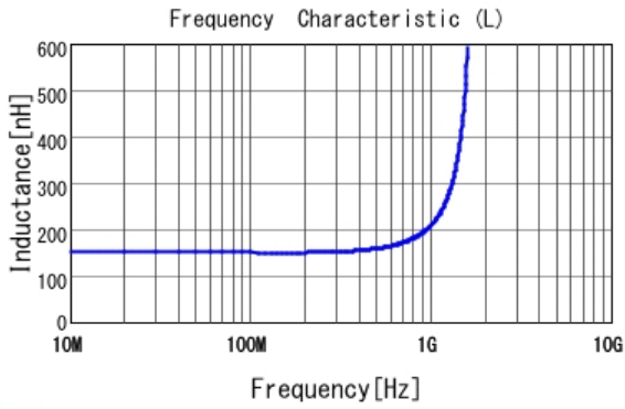
■ LQW18ANR15G00 L
