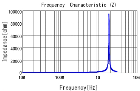
■ LQW18ANR16J00 |Z|
