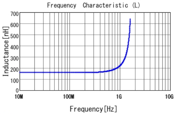
■ LQW18ANR16J00 L
