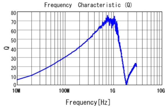
■ LQW18ANR16J00 Q
